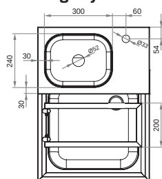
Rzut z góry
