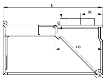
SZCZEGÓŁ A SKALA 1:2
