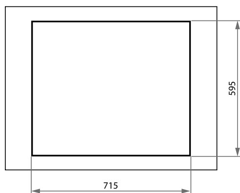
OTWORY MONTAŻOWE WANIEŃ O WYMIARZE 830 X 620 MM
