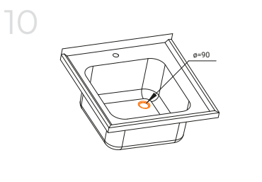
Wycięcie otworu pod młynek
