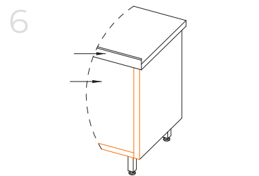
Licowanie tylnej ściany w stole korpusowym
