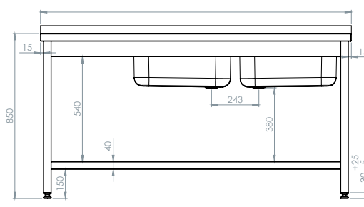
Rzut z przodu
