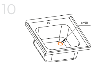
Wycięcie otworu pod młynek
