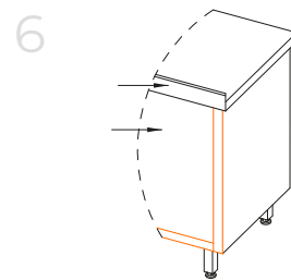
Licowanie tylnej ściany w stole korpusowym
